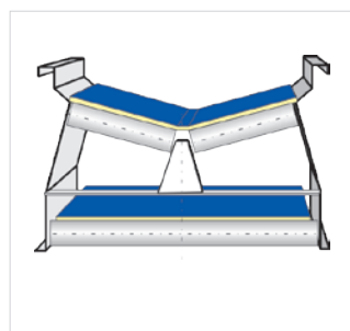
Конструкция RB 500 / RB 650
