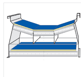
Конструкция RB 800
